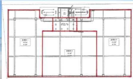
2・3階平面図（分割案）
